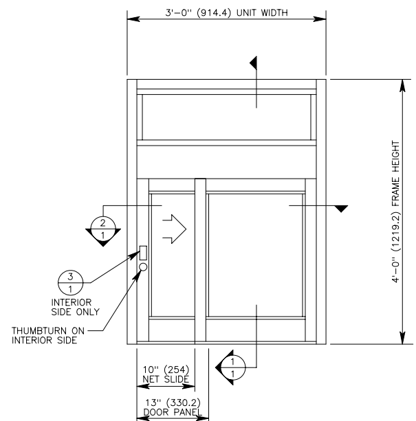
ELEVATION 4 1
