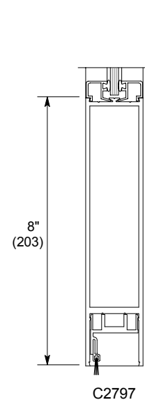
Optional Bottom Rails
