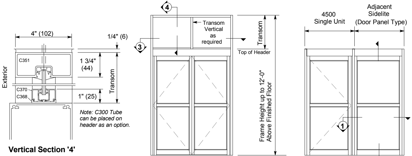
Elevation
